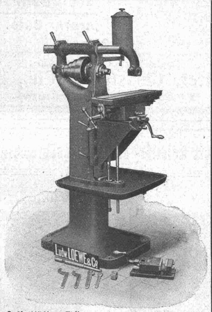
Selbsttätige Fräsmaschine Nr. 12, Modell I.
