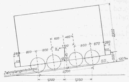
Abb. 39. Schema. — Masstab 1:100.
