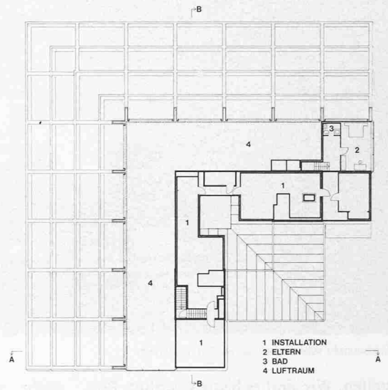
Installationsgeschoss 1:675
