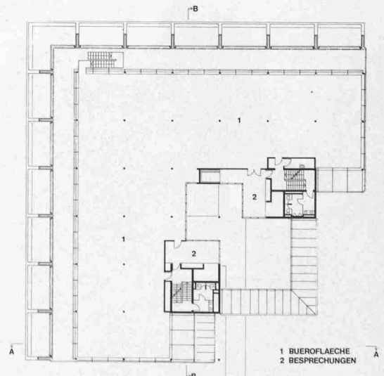
1. Obergeschoss, 1:675
