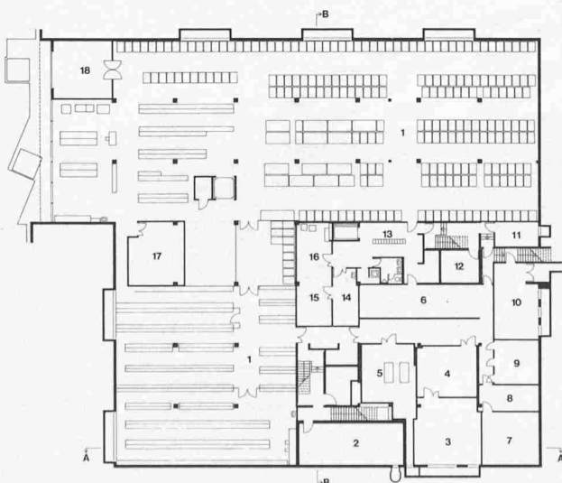
Lagergeschoss, 1:675
