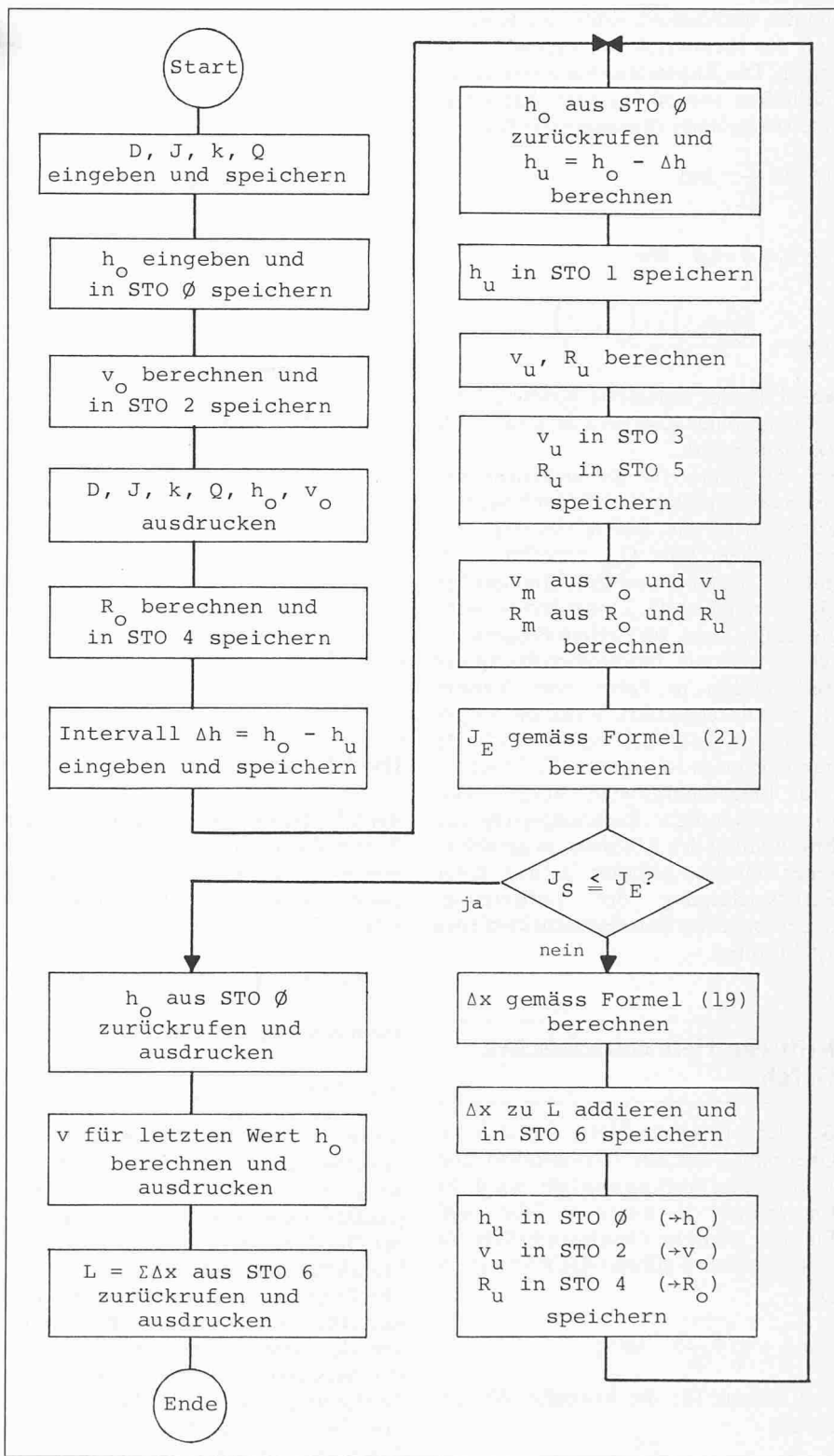
Bild 4. Strukturdiagramm für die Berechnung der Senkungslinie gemäss Formeln (19) und (21) · L = \Sigma \Delta x stellt die Summe der einzelnen um Intervall \Delta h = h_0 - h_u differierten Querschnittsabstände der Rohrleitung dar
