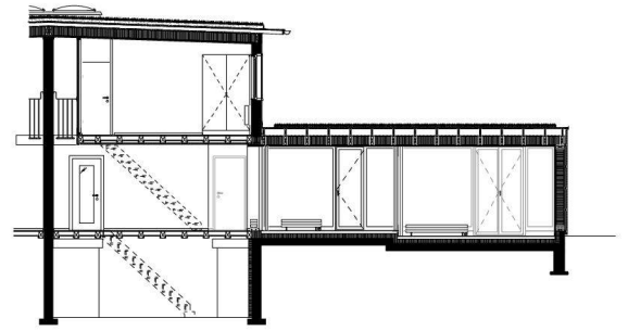
Schnitt A
