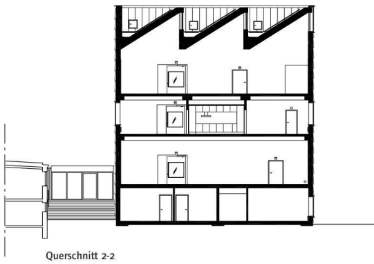
Querschnitt 2-2
