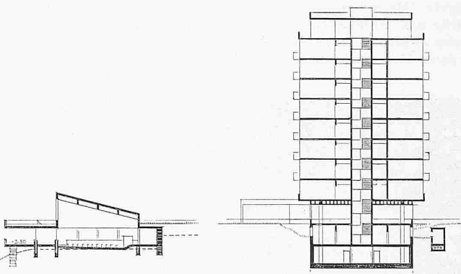
Querschnitt durch Hauptbau 1:800
