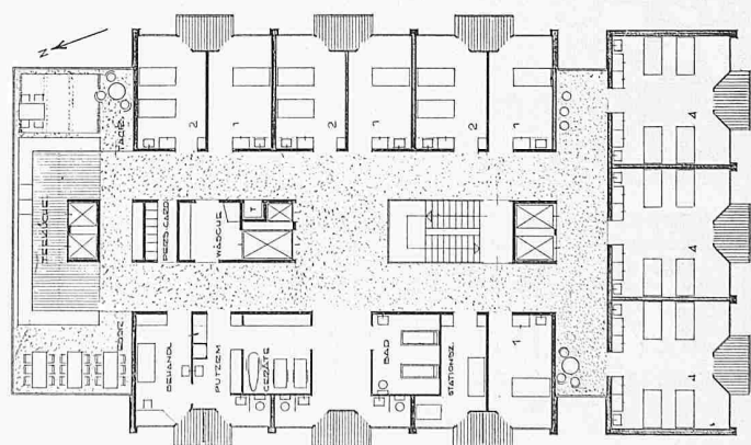
Pflegeeinheit 1:400
