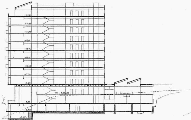
Längsschnitt durch Hauptbau 1:800
