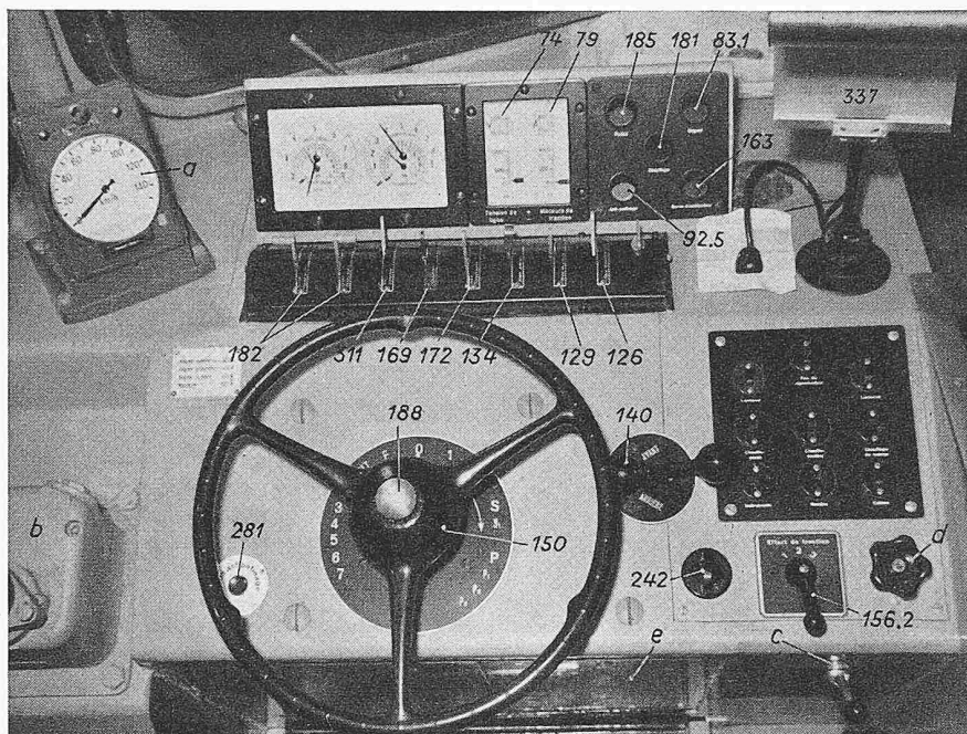
Fig. 10. Vue du pupitre de commande du mécanicien, semblable pour l'automotrice et pour la voiture-pilote
