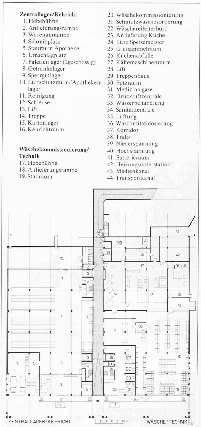
Grundriss 2. Untergeschoss
