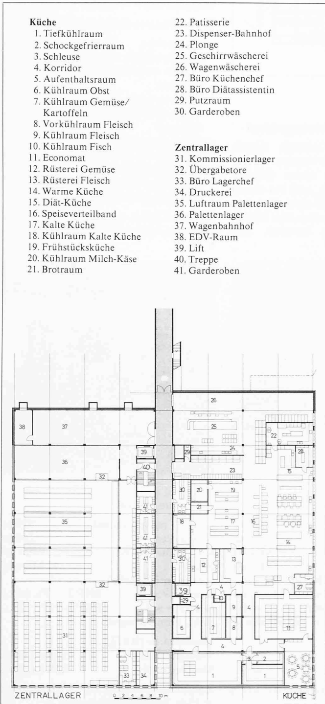
Grundriss 1. Untergeschoss
