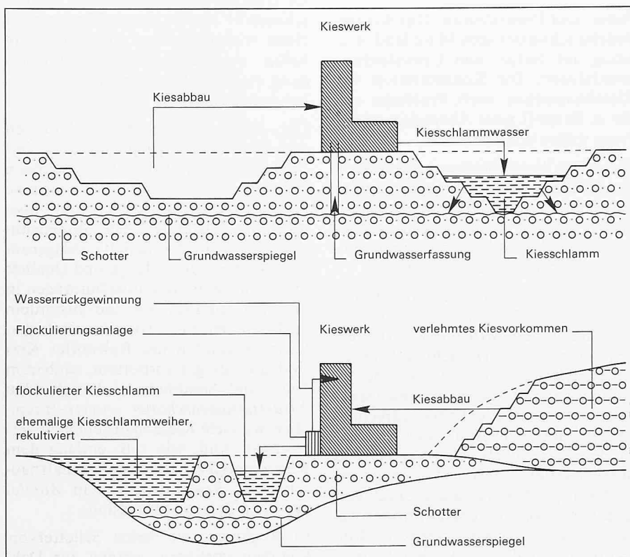
Bild 2. Prinzipschema einer Kiesgewinnung. Oben: Schottervorkommen Unten: Verlehmt Kiesvorkommen
