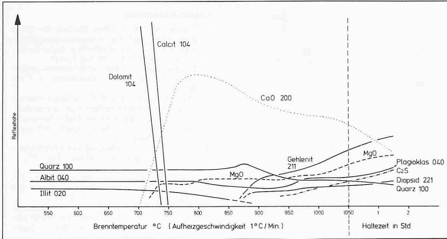
Bild 7. Darstellung des Reaktionsverlaufes der einzelnen Mineralphasen während des Brennens des Kiesschlammtyps G. Aufnahme mit der Röntgendiffraktometer-Heizkamera
