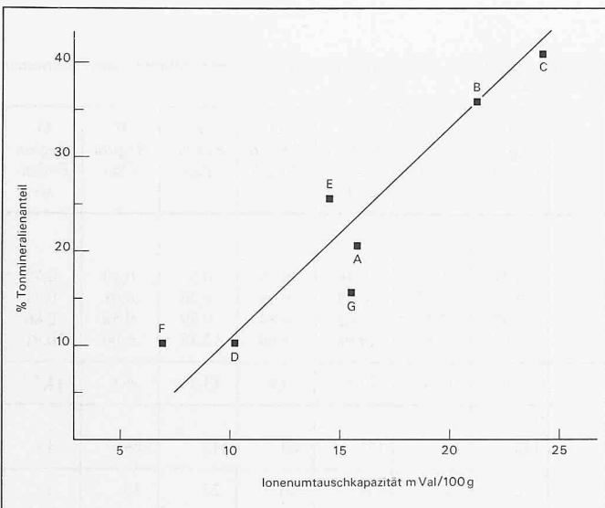
Bild 5. Zusammenhang zwischen Ionenaustauschkapazität und Tonmineralgehalt der Korngrössenfraction <0,063 mm
