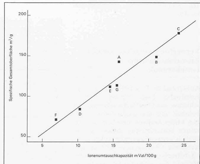
Bild 6. Zusammenhang zwischen Ionenaustauschkapazität und spezifischer Gesamtoberfläche der Korngrössenfraction <0,063 mm
