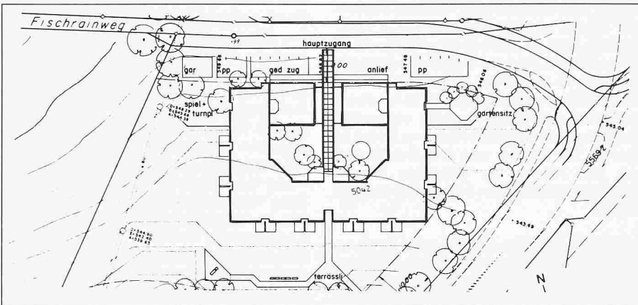
Lageplan 1:1700
