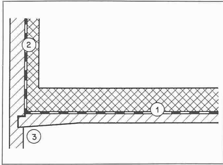
Bild 2. Setzungsfreier Übergang der Bodenplatte zur Baugrubenumschliessung
