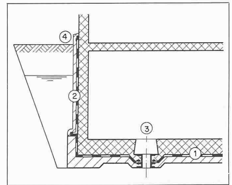
Bild 1. Offene Baugrube und Aussenabdichtung 1 Grundwasserabdichtung horizontal mit Schutz- schicht 2 Grundwasserabdichtung vertikal, Aussenabdich- tung mit Schutzschicht, angeschlossen mit rück- läufigem Stoss 3 Grundwasserentlastungsstutzen mit Pumpen- sumpf 4 Anschluss an Gebäude, mind. 0,15 m über Terrain
