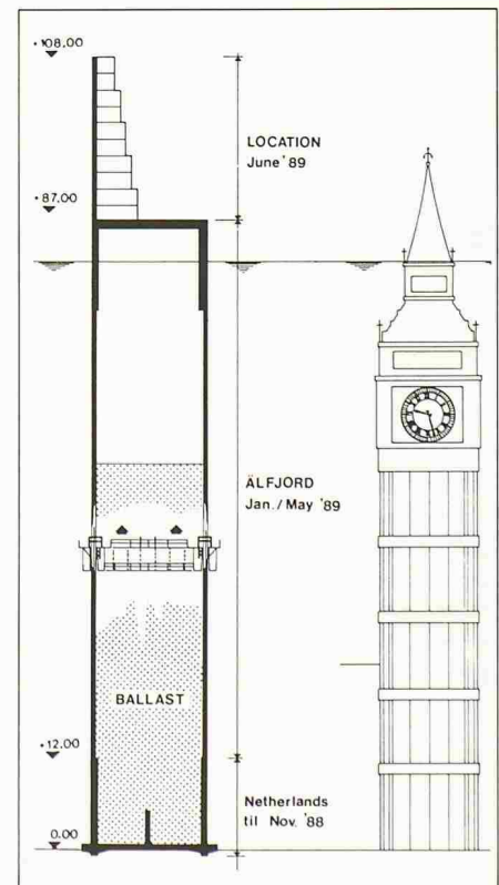
Bild 5. Querschnitt der Schutzwand von Bild 3 mit Bauabschnitten und Vergleichsgebäude
