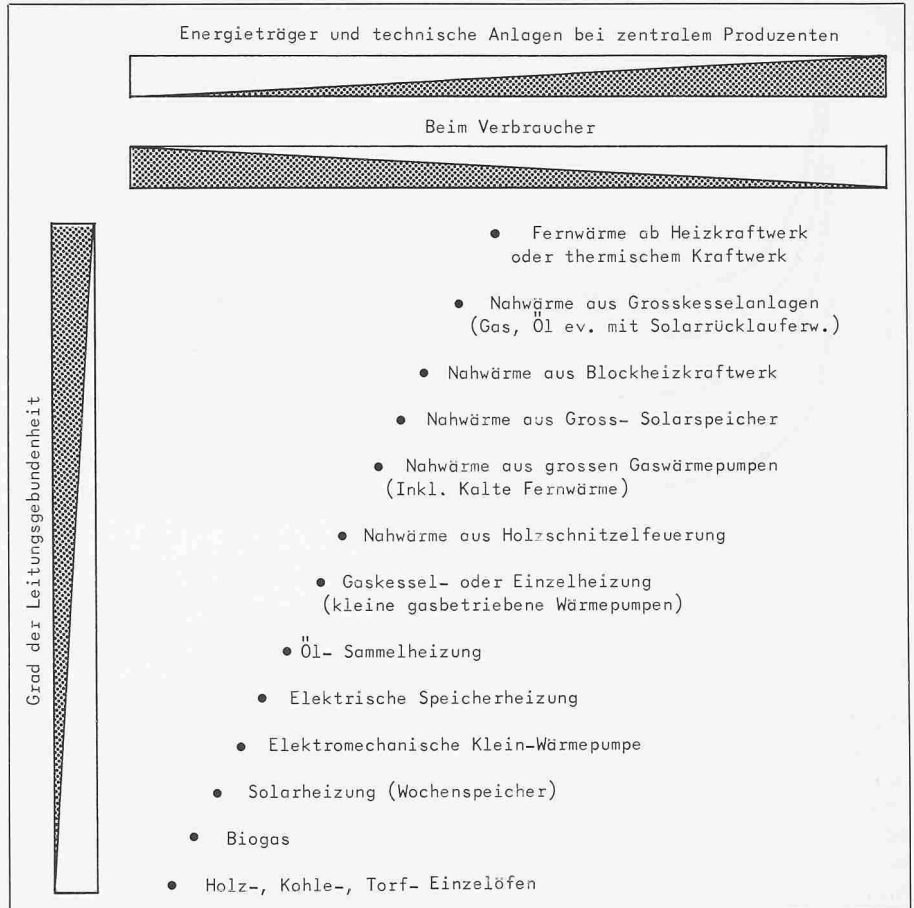
Bild 11. Untersuchte Wärmeversorgungssysteme
