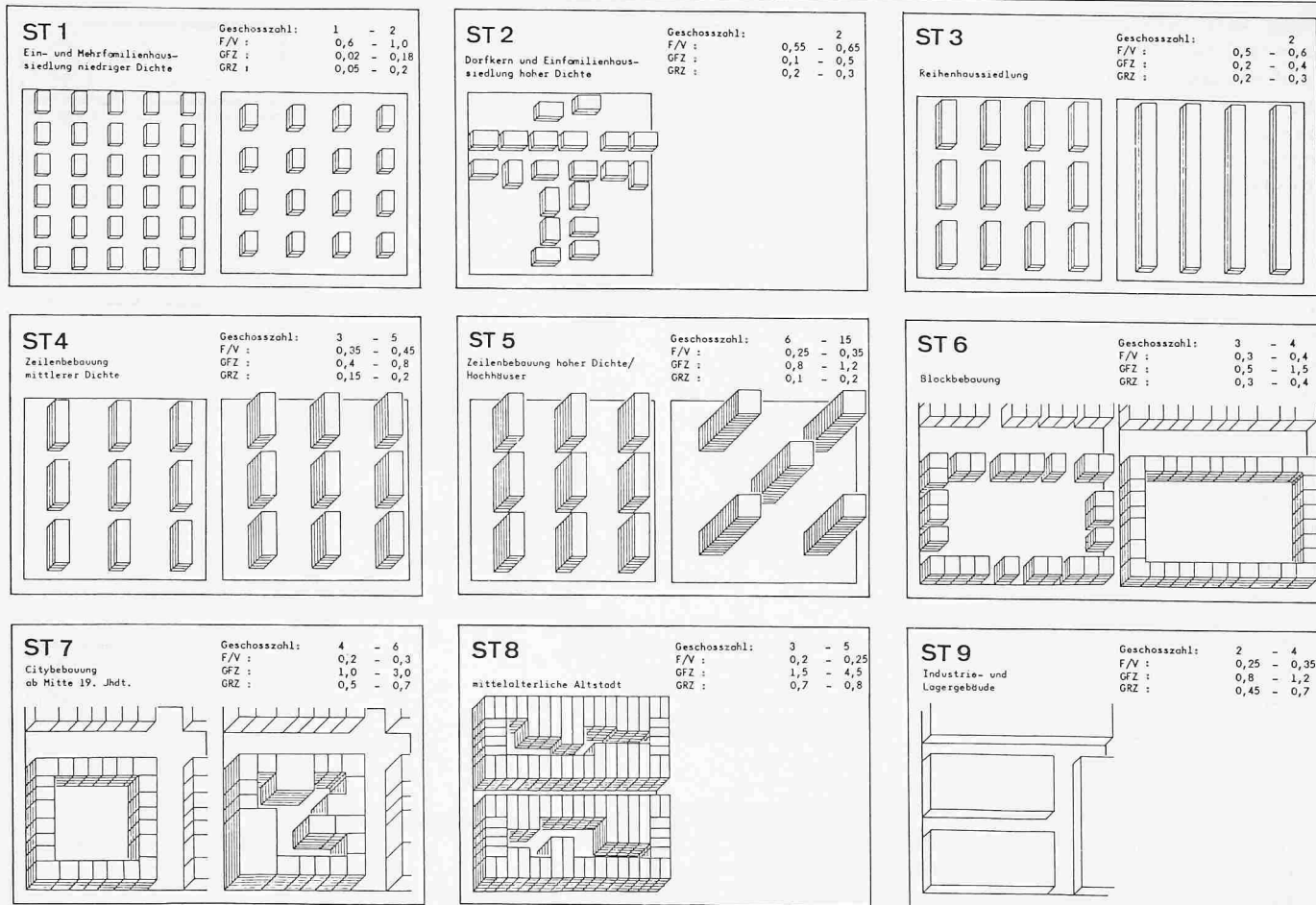
Bild 4. Siedlungstypenmodell, Übersicht
