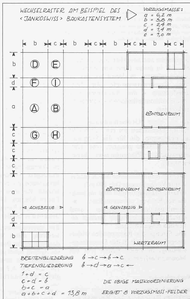
Bild 9. Aufbau eines Wechslerrasters für Röntgenabteilung
