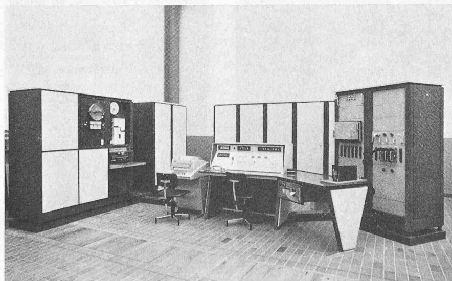
Bild 2. Gesamtansicht des Automated Test Equipment Complex (ATEC) der Swissair. Links der Digital-Computer CDC 1700, daneben die Programmierstation (Fernschreiber und Lochstreifenstanzer), im Hintergrund links das «Interface»-Gerät (Übersetzungselektronik zwischen Digital-Computer und der mit analogen Signalen arbeitenden Prüfstation), in der Mitte die Bedienungs- und Überwachungskonsole und rechts die eigentliche Prüfstation. Diese umfasst die fünfteilige Anlage mit den Spannungsquellen, Simulatoren und Messeinrichtungen (Hintergrund), die zweiteilige Anschlusseinheit (rechts), an der der Prüfling (auf dem Tisch) angeschlossen wird. Unter dem Tisch ist der das Prüfprotokoll druckende Apparat sichtbar
