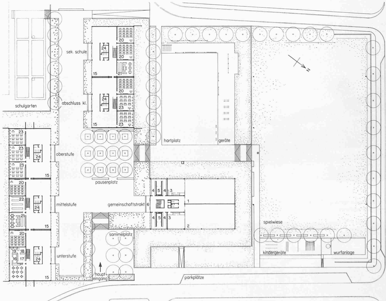
Erdgeschoss 1:1100
