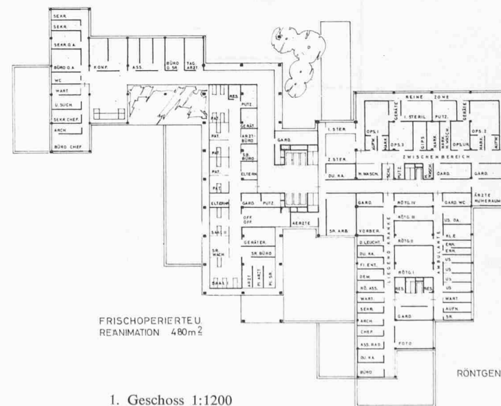
1. Geschoss 1:1200
