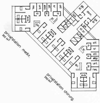
Geschoss i 1:1200
