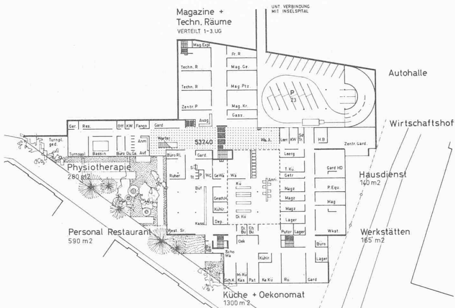
2. Untergeschoss 1:1200
