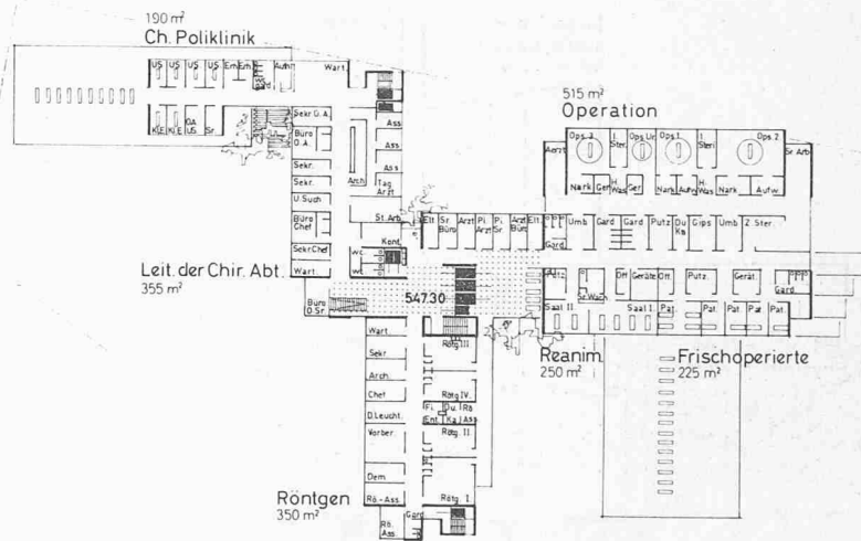
1. Geschoss 1:200
