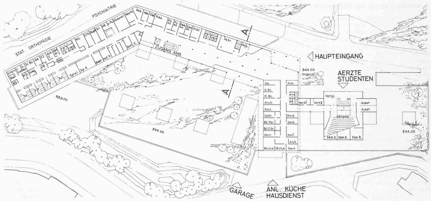
Erdgeschoss 1:1200
