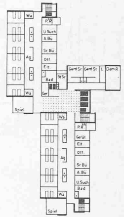
9., 8., 7., 6. Gesch. 1:1200
