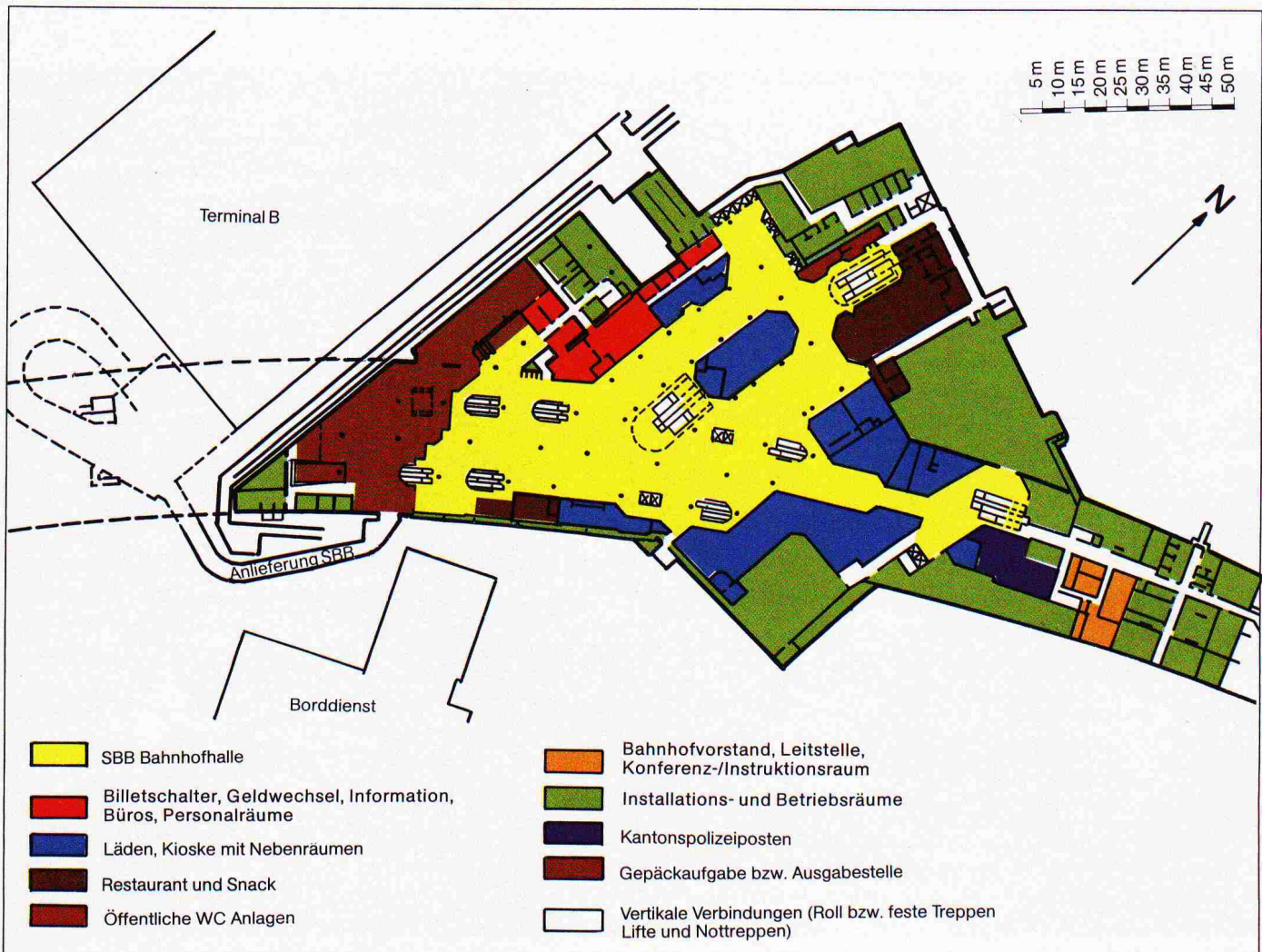
Bild 4. Bahnhofhalle. Grundriss
