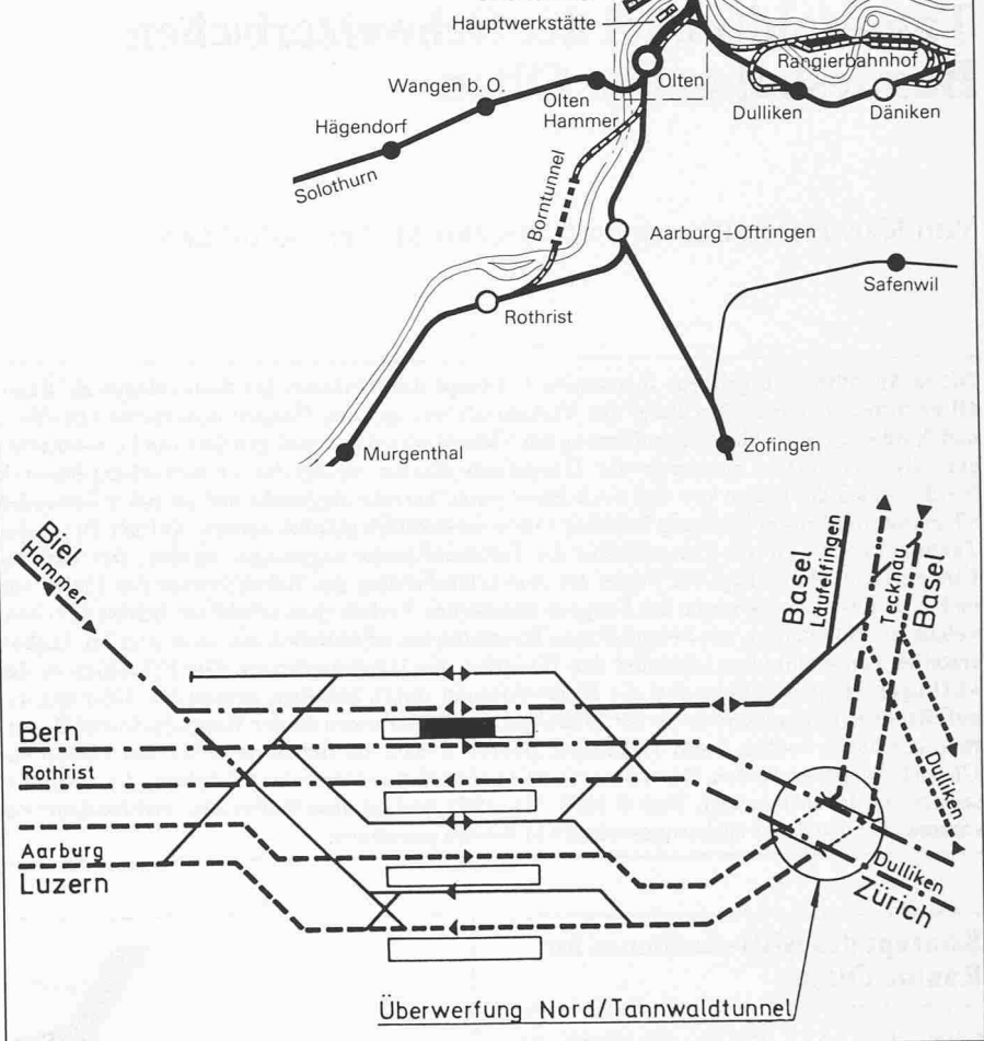
Bild 3. Übersicht über die 1. Etappe der Entflechtung der Verkehrsströme im Raum Olten. Verlauf der Bahnlinien im Bereich des Bahnhofes Olten (gestricheltes Rechteck) gemäss untenstehendem Schema
