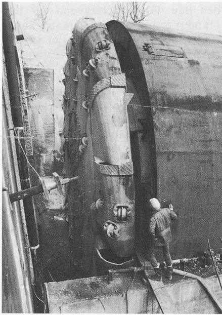
Bild 8. Vollschnittfräse
