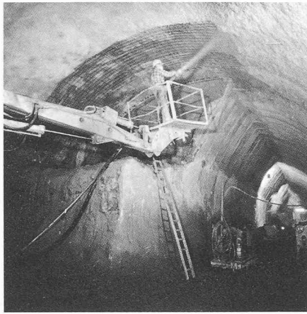
Bild 16. Spritzbetoneinbau im Firstbereich im Tunnelbau
