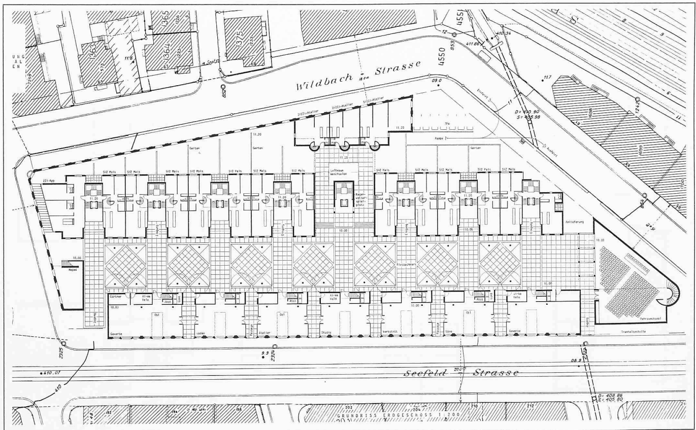
Grundriss Erdgeschoss 1:1000
