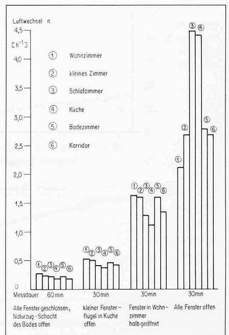
Bild 3. Messresultate für den Luftwechsel in den verschiedenen Räumen einer Wohnung ( t_{\text{aussen}} um -1 \text{ }^\circ\text{C} ; Windgeschwindigkeit etwa 6,5 \text{ m/s} )
