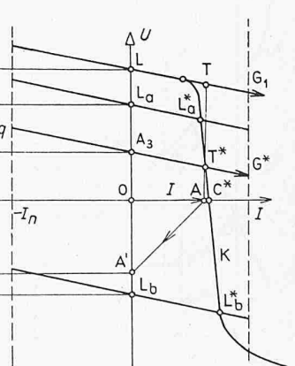
Bild 13b. Äussere Kennlinie K bei Gegenkopplung
