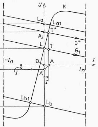
Bild 10b. Äussere Kennlinien K bei Mitkopplung. Linearer Bereich L_{a1} L_{b1}
