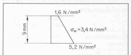
Bild 7. Gesamtverformungen: Spannungsüberlagerung von Bild 5 und Bild 6
