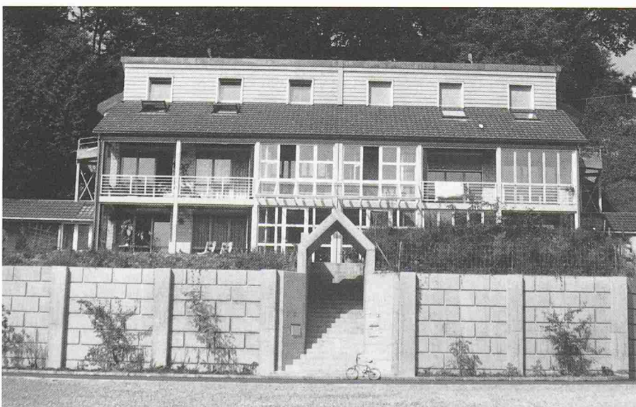
Bild 3. Doppelseitenhaus in Wald. Die nordseitig erdbedeckten Doppelwohnhäuser mit gemeinsamen Zugang sind auf der ganzen Südfront mit verglasten zweigeschossigen Veranden ausgeführt, welche im Sommer zurückgeklappt werden können. Die Solarbauten in Wald sind tief ins Erdreich eingebettet. Die innere Vertikalzonierung (thermische Schichtung) ist von aussen ablesbar. Die verglasten Veranden sind im Sommer Balkone resp. Sitzplätze
