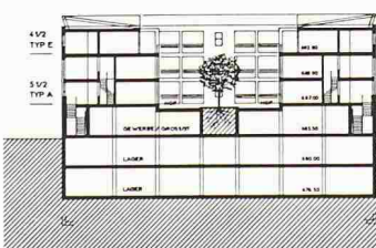
Längsschnitt A-A
