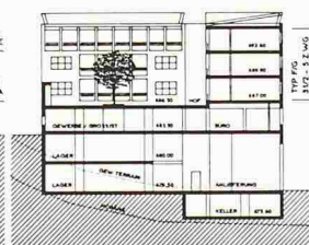
Querschnitt B-B
