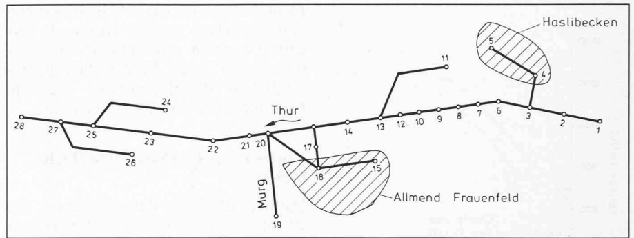
Bild 4. Aufteilung der Berechnungsstrecke in Flussäste und Knoten für das Richtprojekt 1979; Knoten 1: oberes Ende der Berechnungsstrecke bei TG km 23.930, Knoten 19: Murg bei der hydrometrischen Station Frauenfeld, Knoten 20: Zusammenfluss von Murg und Thur, Knoten 28: unteres Ende der Berechnungsstrecke bei ZH km 14.800 (2,3 km unterhalb TG km 0.000)
