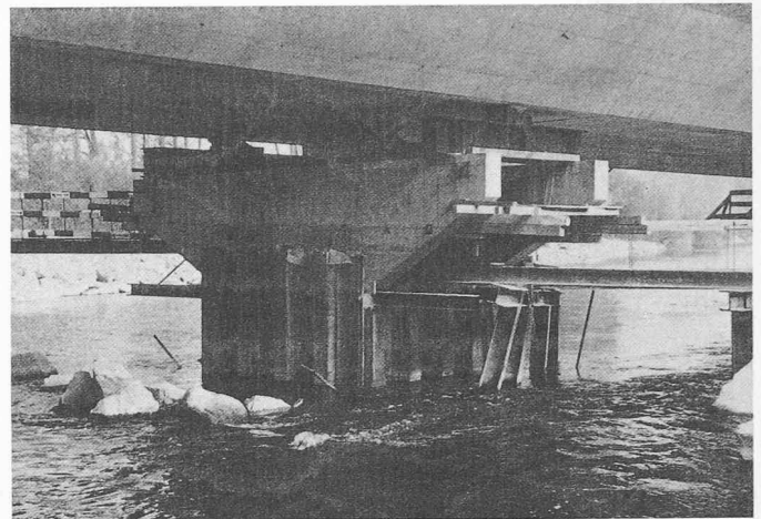
Bild 11. Pfeiler 2 mit provisorischen seitlichen Stabilisierungsstützen
