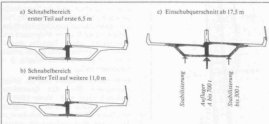
Bild 9. Vorbauschub als Brückenteil (Querschnitte)
