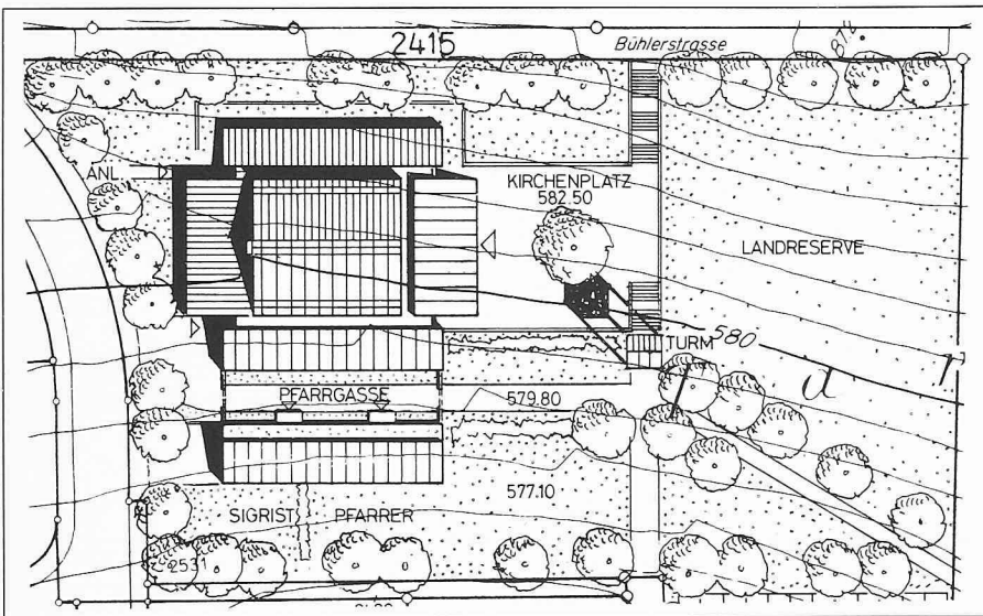
Lageplan 1: 1000
