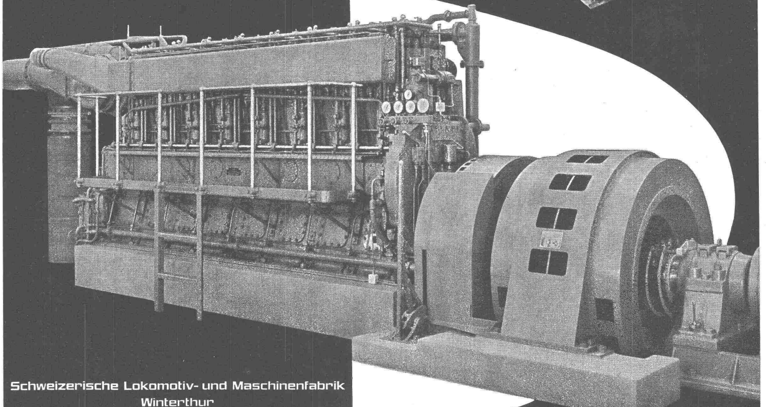
750 kW Notstromgruppe
