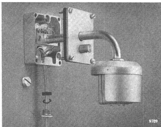
Aussenfühler der Zentralheizungsregulierung «Sigma» mit abgeschraubter Deckplatte. Das angeschlossene Kabel kann auch direkt in die Mauer verlegt werden. Auf der Vorderseite der Deckplatte ist der Belüftungsstutzen sichtbar.
