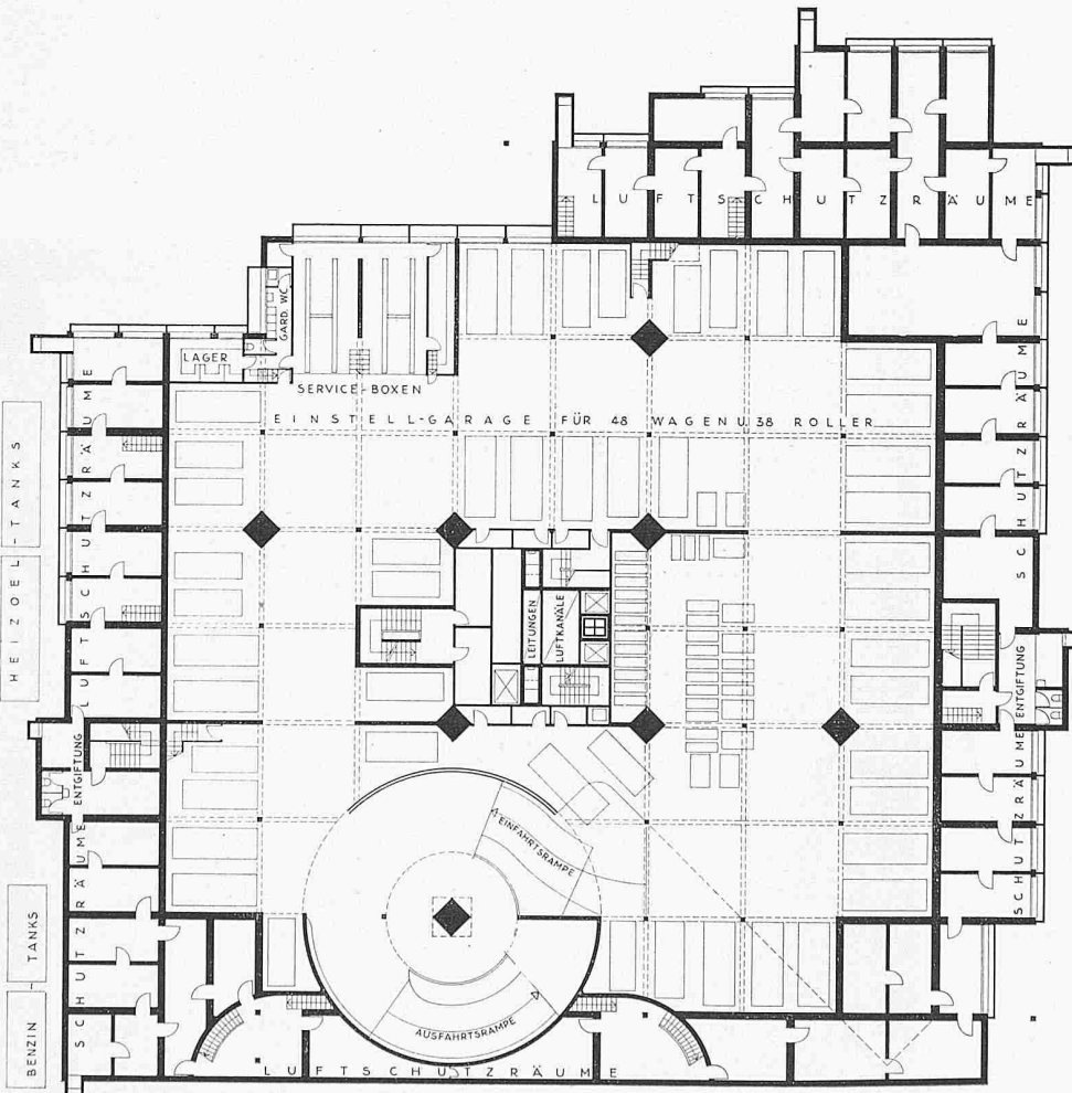
7 Schnitt A-A, 1:500
