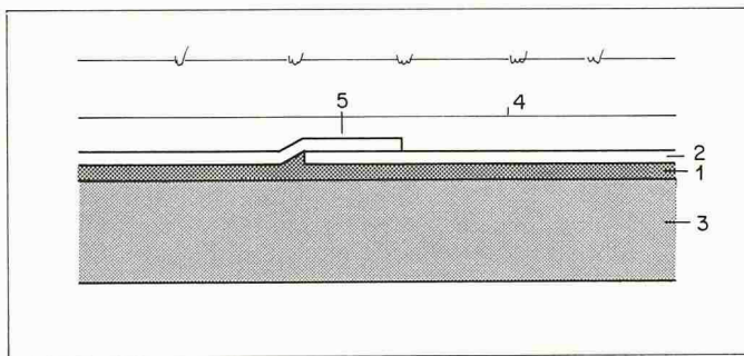
Bild 3. Vollflächige Verklebung von Kunststoffdichtungsbahnen. (1) Hohlräumfüllender Kleber, z.B. Zweikomponenten-PU; (2) Kunststoffdichtungsbahn; (3) Betondecke/Wand; (4) Schutzschicht (z.B. Schuttmörtel oder Schutzmatte); (5) Stösse überlappt oder stumpf mit Bandschweissen.
