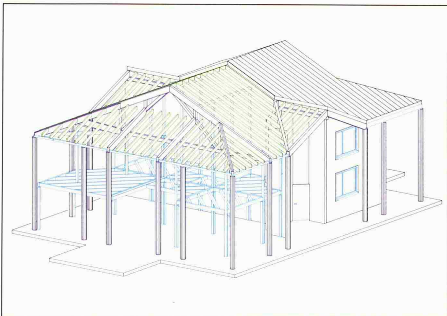
Bild 1. Tüffeln: Axonometrie einer Holzkonstruktion. Architekten: Schär, Port und Sommer; Ingenieure: Bois-Consult Natterer SA, Etoy
