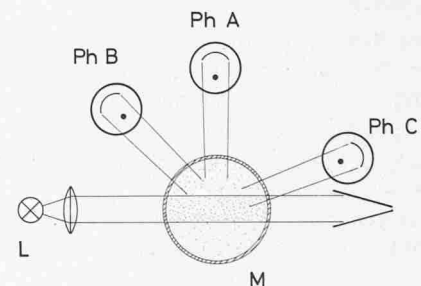
Bild 2. Prinzip der Streulichtmessung
