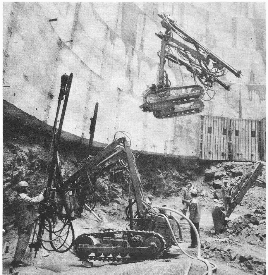
Bild 10. Abteufen des 82 m tiefen Schachtes für das Kraftwerk Kühltai; Felswand unter der Betonauskleidung 3,00 m hoch freistehend
