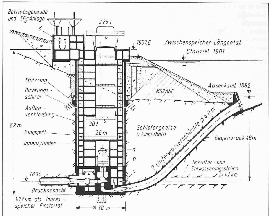
Bild 9. Als Schachtkraftwerk ausgeführtes Pumpspeicherwerk Kühltai mit zwei Maschinensätzen (247 MW Motor- oder Pumpleistung und 286 MW Generatorleistung) für die Kraftwerkgruppe Sellrain-Silz. Längsschnitt
