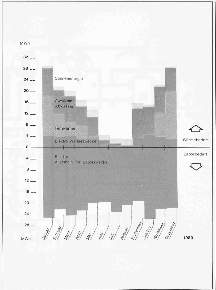
Bild 3. Monatlicher Energieverbrauch im Kantonalen Chemischen Laboratorium
