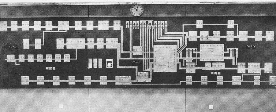
Bild 2. Fahrleitungsfernsteuertafel im UW Olten
