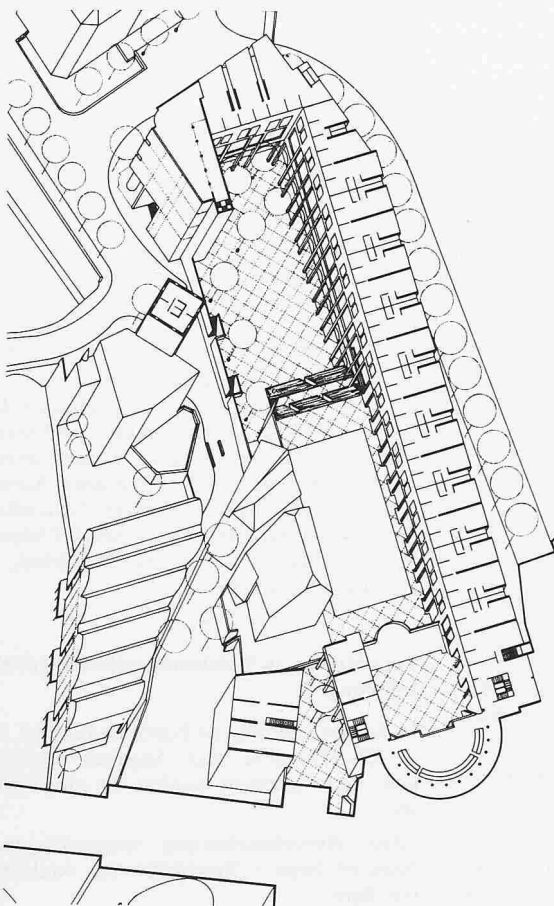
Grundriss Ebene 517.40, 1:1500
