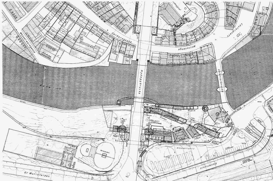
Lageplan 1:2700
