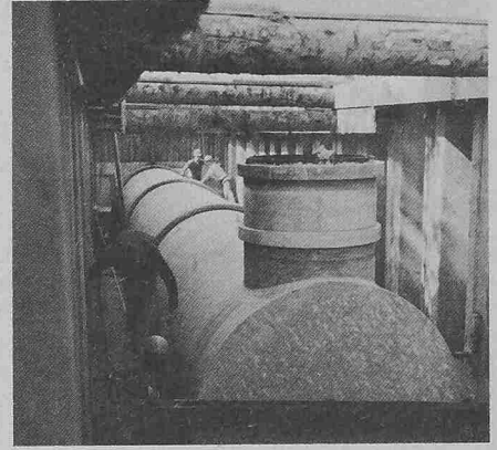
Das Abschlusselement mit Einstiegsdom ist montiert
