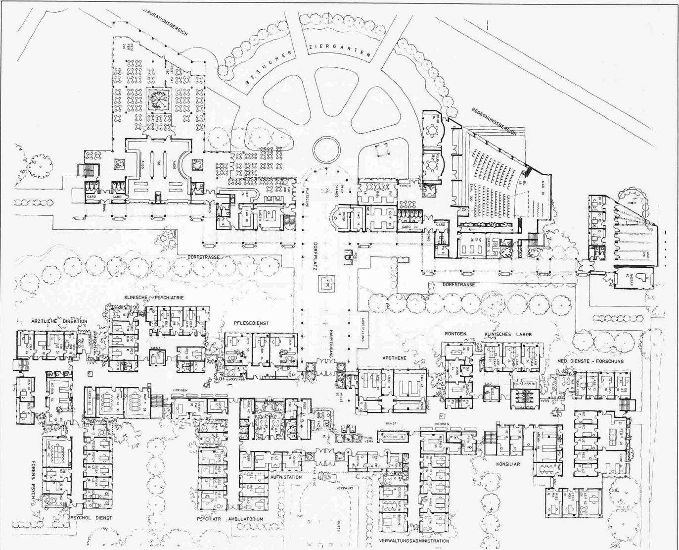
Grundriss Erdgeschoss 1:800
