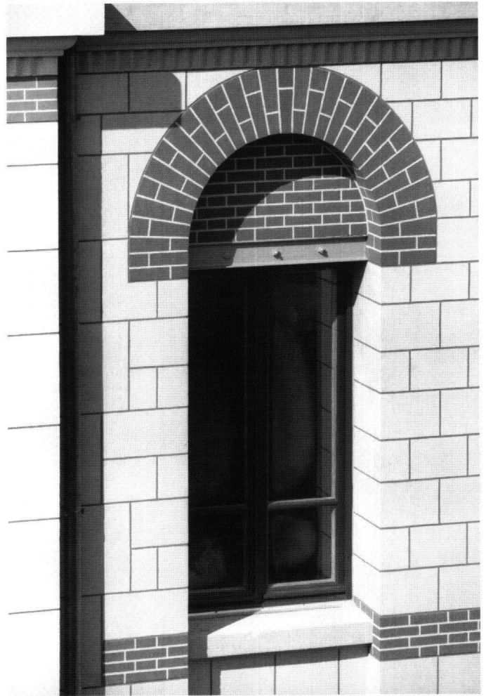
Abb. 17: Küssnacht, Gymnasium Immensee , «Z-Bau», Fassadensanierung. Bei den hellen Quadern ist der Grundputz dunkel, bei den ziegelroten Quadern hell eingefärbt. Gut zu erkennen sind der metallene Fenstersturz sowie die rot lasierten originalen Fenster.
