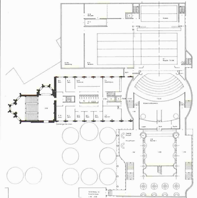
Parkett/Bühnengeschoß
