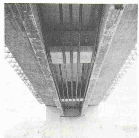
Bild 4. Doppelstegiger Plattenbalken mit aussenliegenden Spanngliedern ohne Verbund teilweise vorgespannt (Franz/Miessler)
