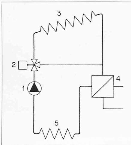
Kombination Luftregister/Erddollektor 1 Umwälzpumpe 2 Verteilventil 3 Luftregister Carport 4 Verdampfer, Wärmepumpe 5 Erdollektor
