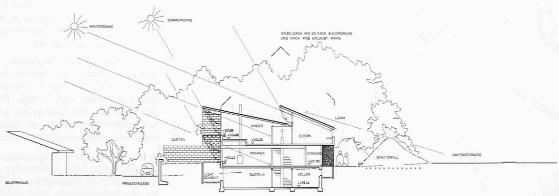
Schnitt
