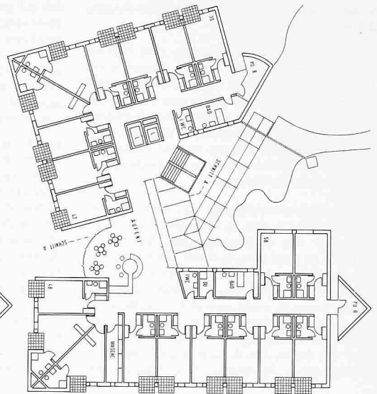
Grundriss 2. Obergeschoss 1:600
