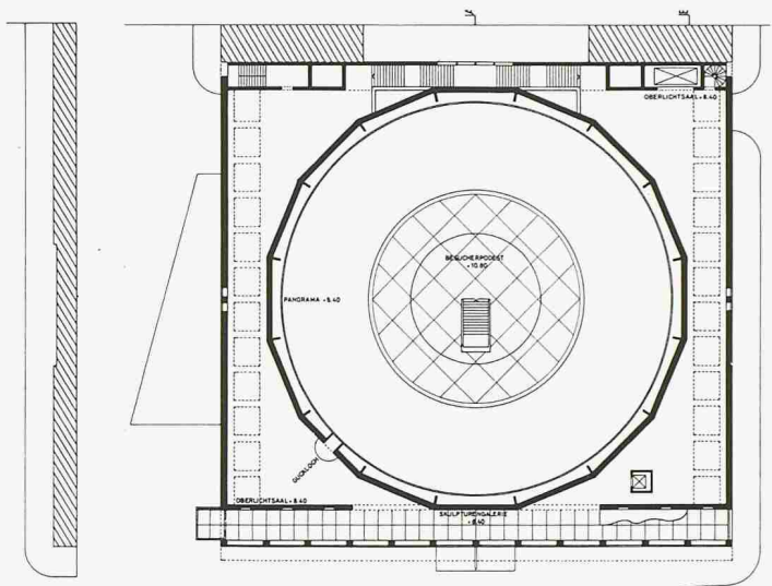
2. Obergeschoss
