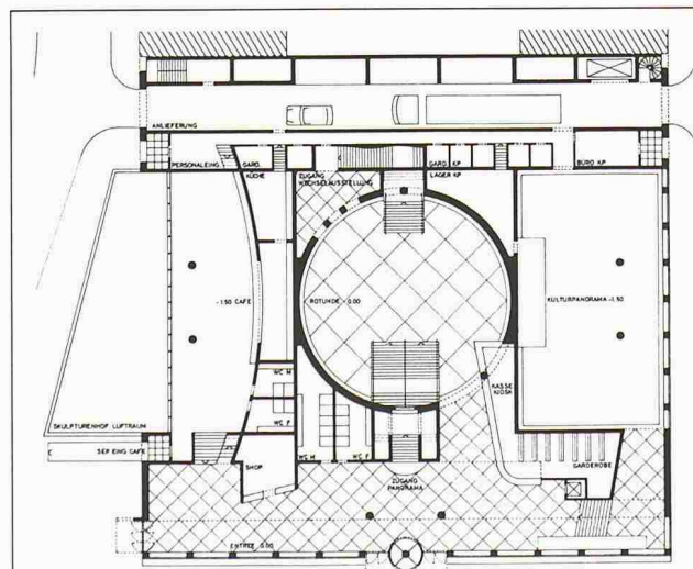
Erdgeschoss 1:550
