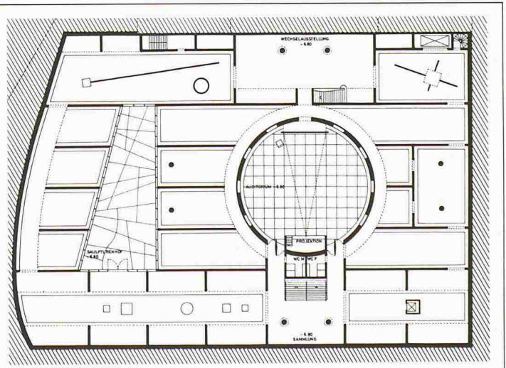
1. Untergeschoss
