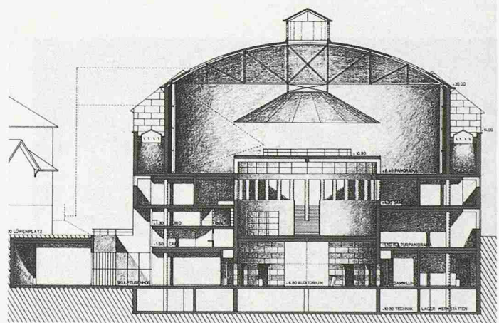
Schnitt C
