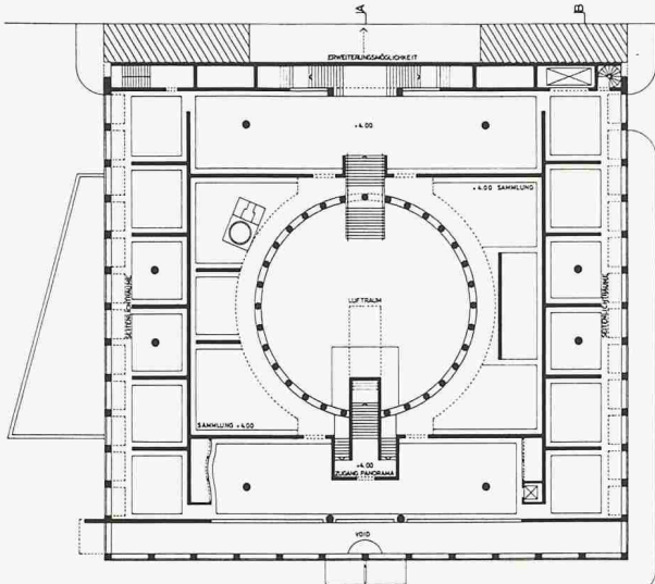
1. Obergeschoss
