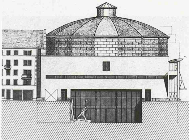
Nordfassade
