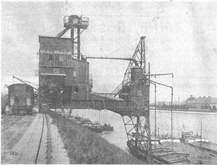
Pneumatischer Getreideheber, Bauart Bühler, für eine Stundenleistung von 70 bis 80,000 kg Weizen, geliefert für das Schifffahrtsamt des Kantons Basel-Stadt für den Rheinhafen Basel-St. Johann
